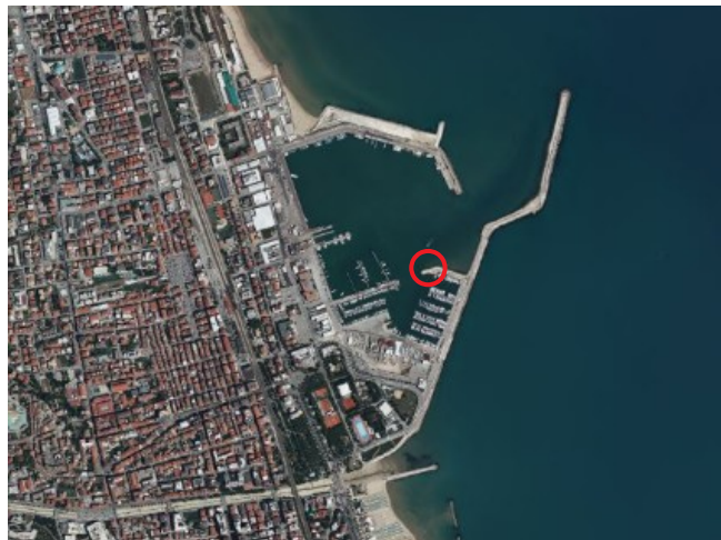
Foto aerea
